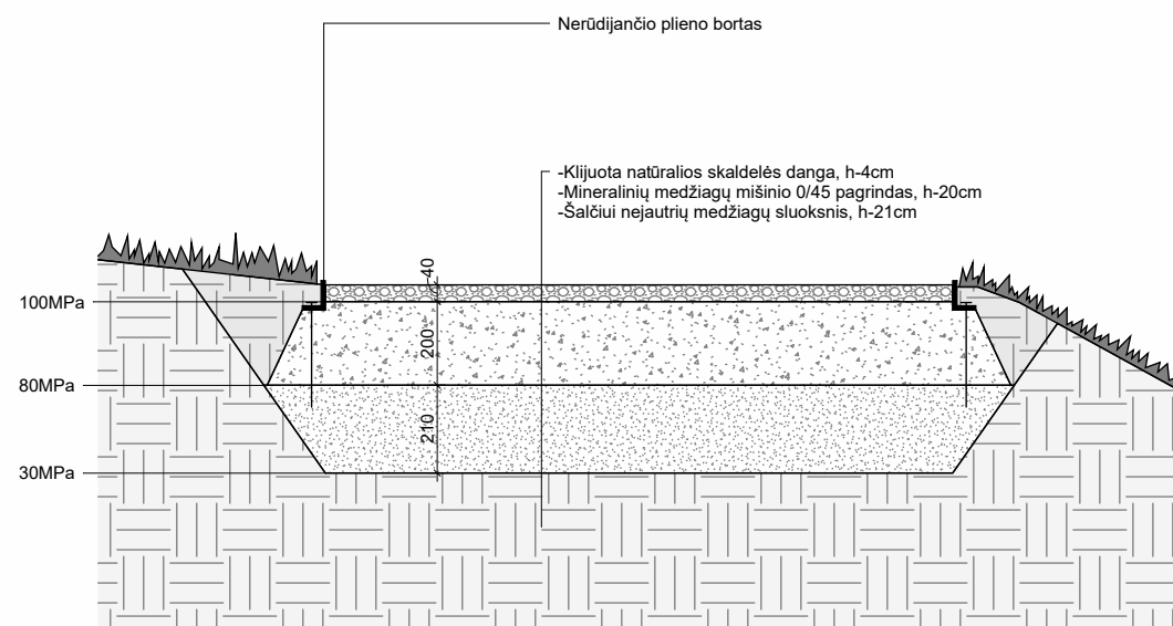
Detailė A 1 : 20
