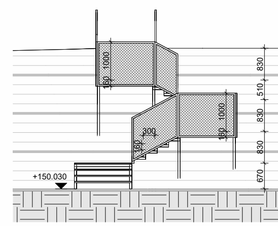
Laiptų "D" Vaizdas iš priekio 1 : 100
