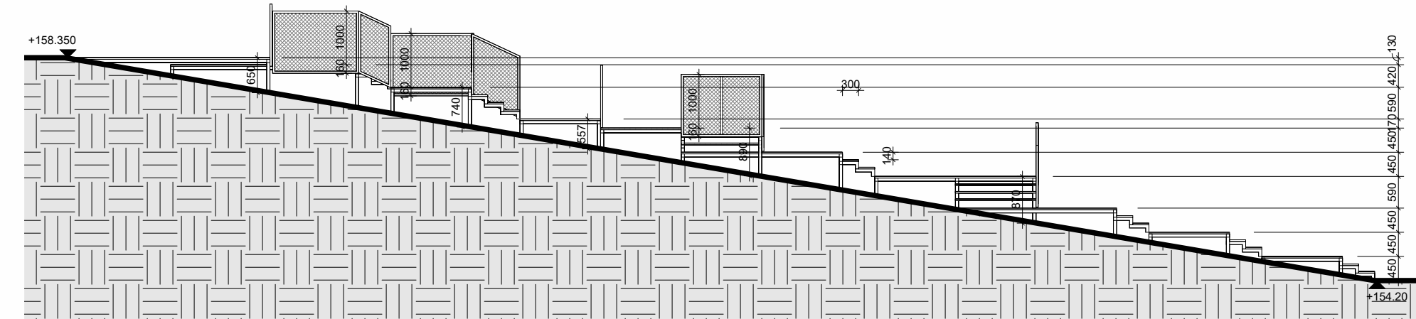
Laiptų "C" Vaizdas iš šono 1 : 100
