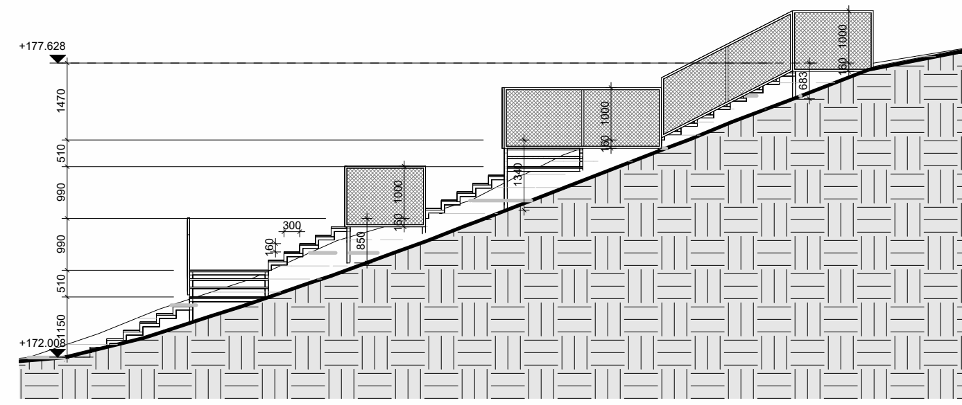
Laiptų "A" Vaizdas iš šono 1 : 100
