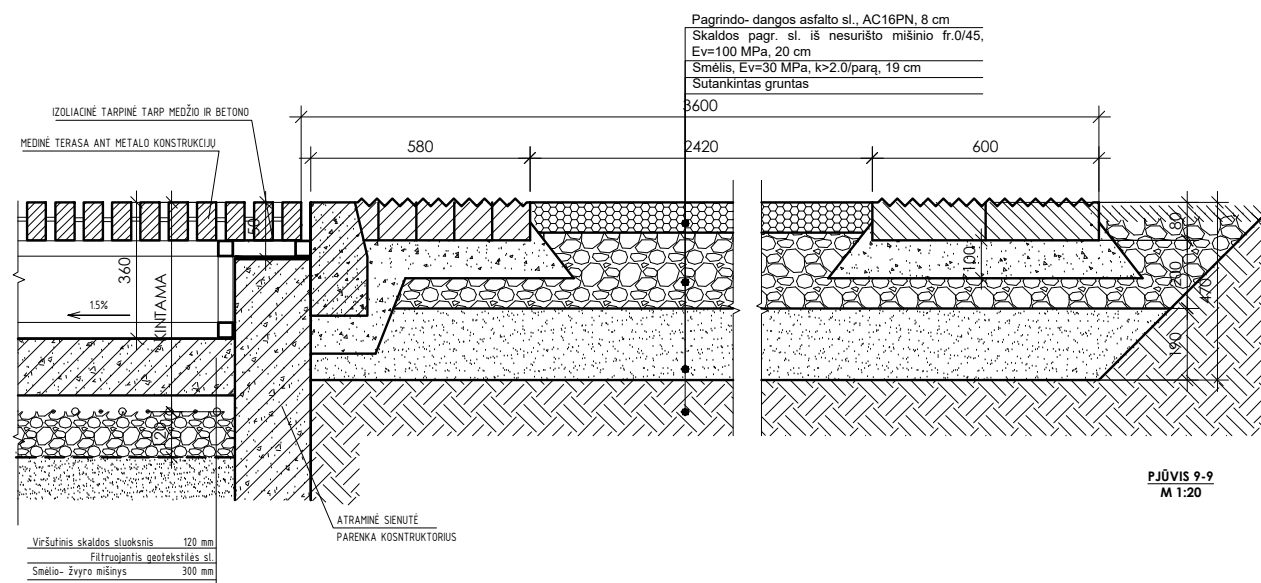
PJŪVIS 8-8 M 1:20
