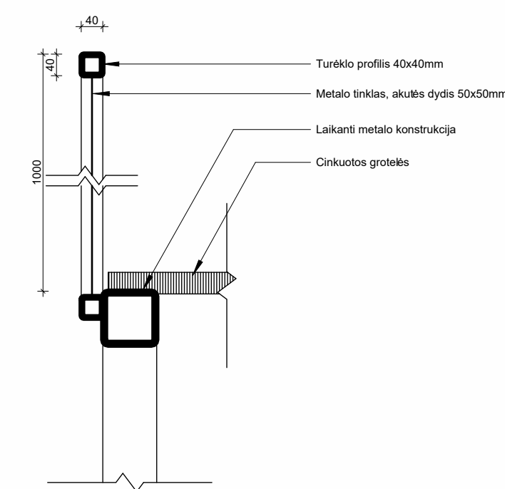
Principinė detalė 1 : 10
