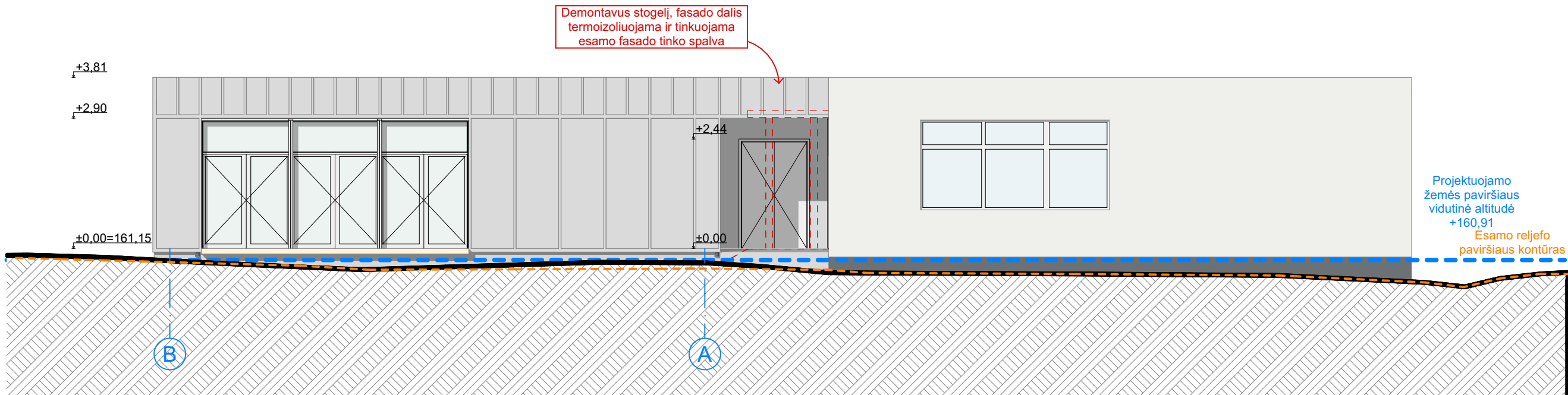
1-2 PIETVAKARINIS FASADAS 1:100
